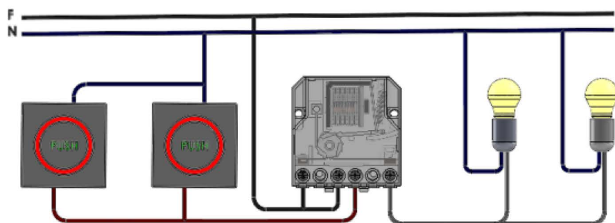
Schema collegamento 1 contatto 1 contact wiring diagram 25040
