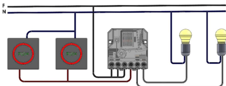
Schema collegamento 2 contatti 2 contacts wiring diagram 25041
